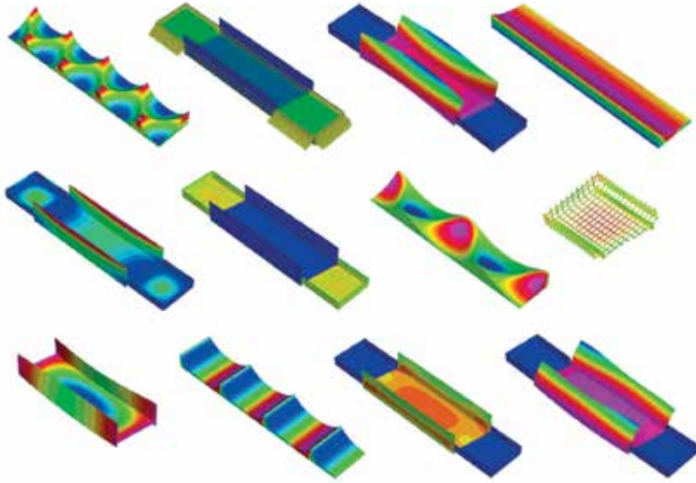
Havuz yapısının doğal frekanslarının ve su çalkalama frekanslarının analizi
